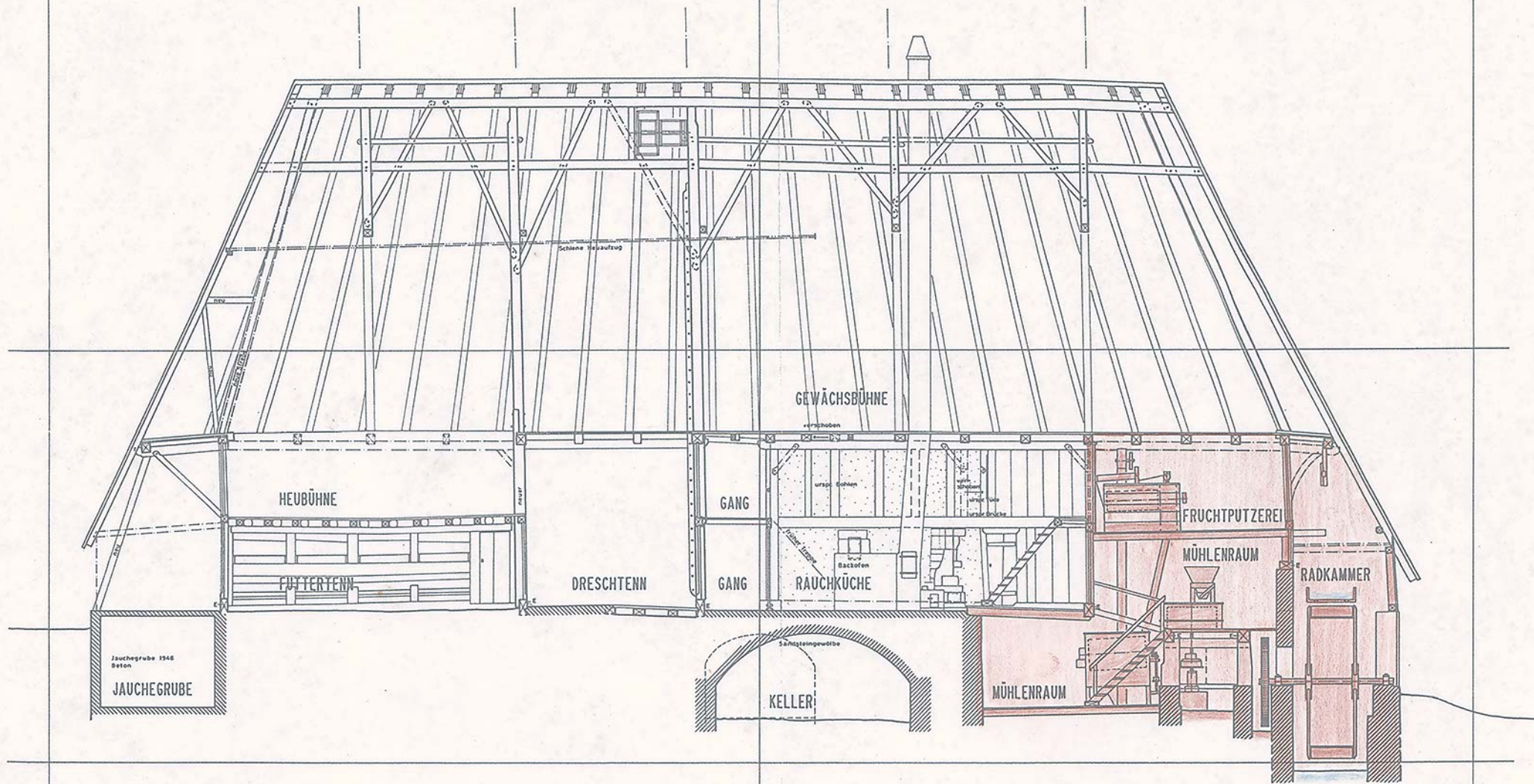
LÄNGSSCHNITT A - A
